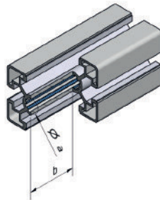
GEWINDE IN ALLEN KERNZÜGEN [Z]
