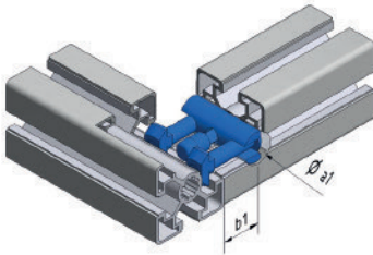
BOLZEN- UND SCHNELLSPANNVERBINDER [D]
