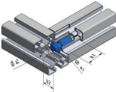
SCHRAUBVERBINDUNG [D]
