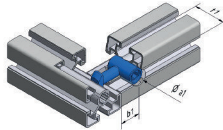
SCHNELLSPANNVERBINDER [DB]
